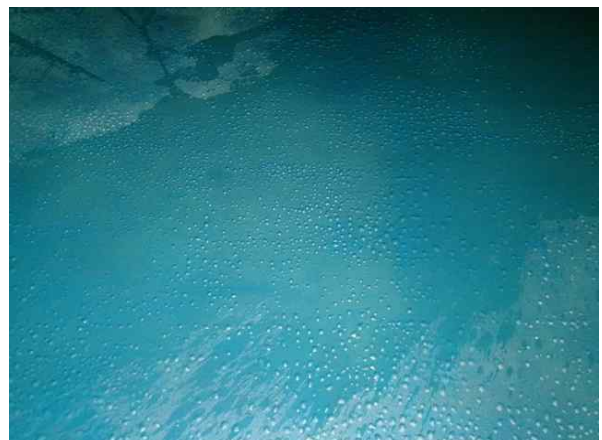
<배수지 1지 바닥슬래브 도장기포>
